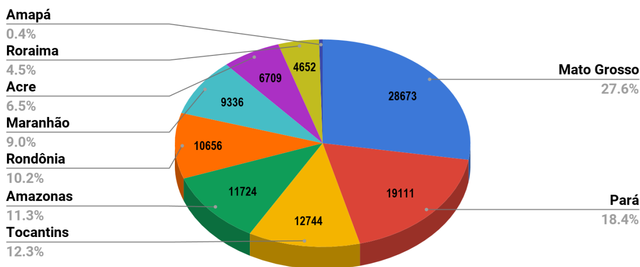
Figura 1 – Distribuição percentual dos focos de queimadas acumulados em 01/01/2019 a 20/10/2019 na Amazônia legal ( Satélite de Referência AQUA Tarde)
