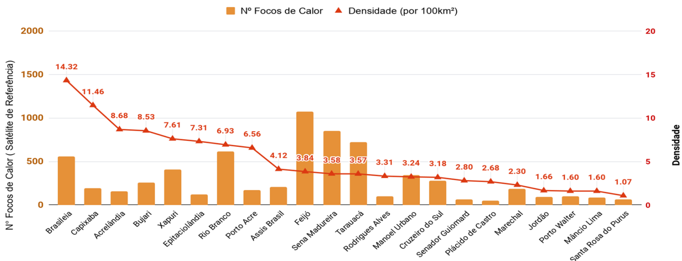
Figura 6 – Ocorrência de focos de queimadas e densidade por km 2 , por município em 01/01/2019 a 20/10/2019 ( Satélite de referência AQUA TARDE)
