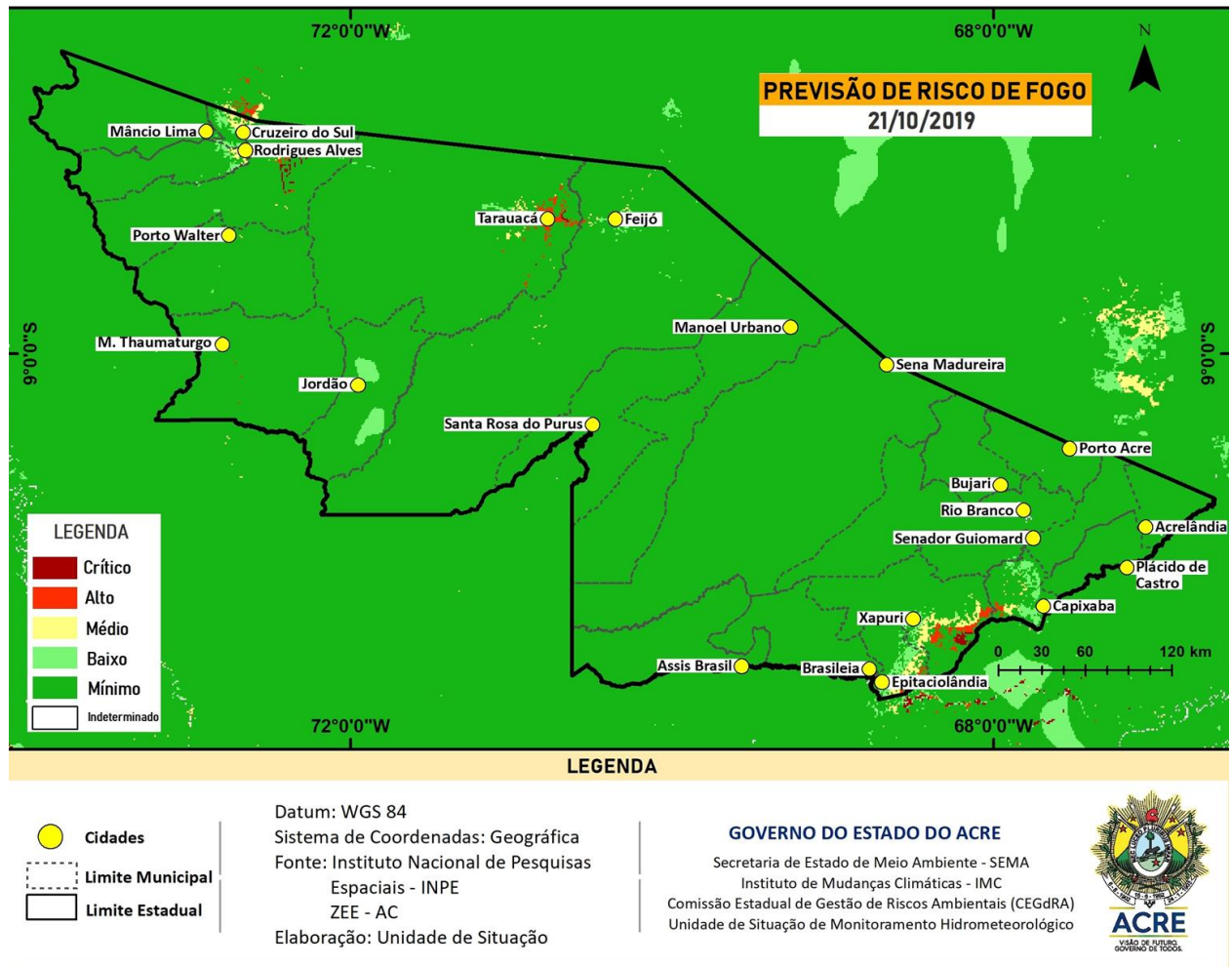
Figura 9 – Risco de Fogo para o estado do Acre em 21/10/2019
