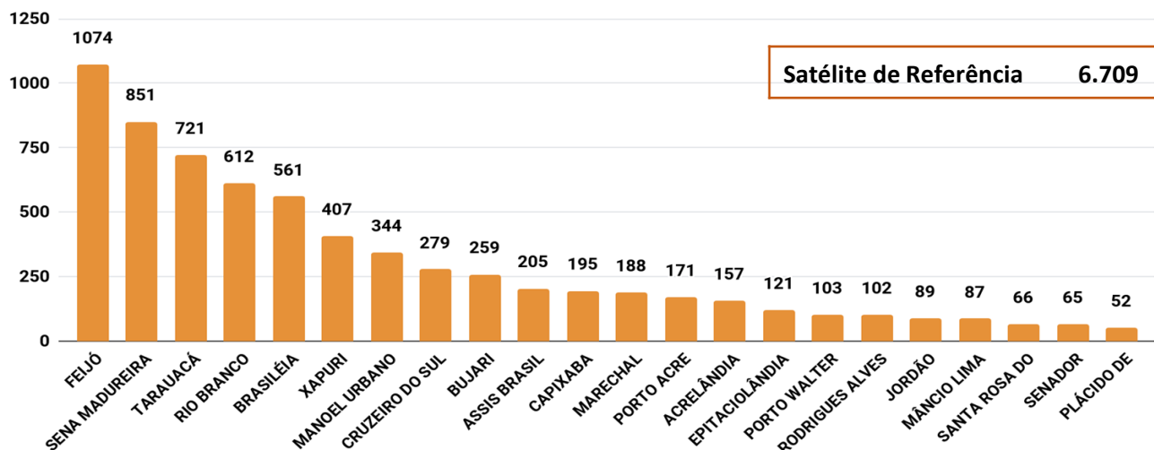
Figura 3 – Distribuição dos focos de queimadas acumulados de 01/01/2019 a 20/10/2019, no Estado do Acre. ( Satélite de referência AQUA TARDE)
