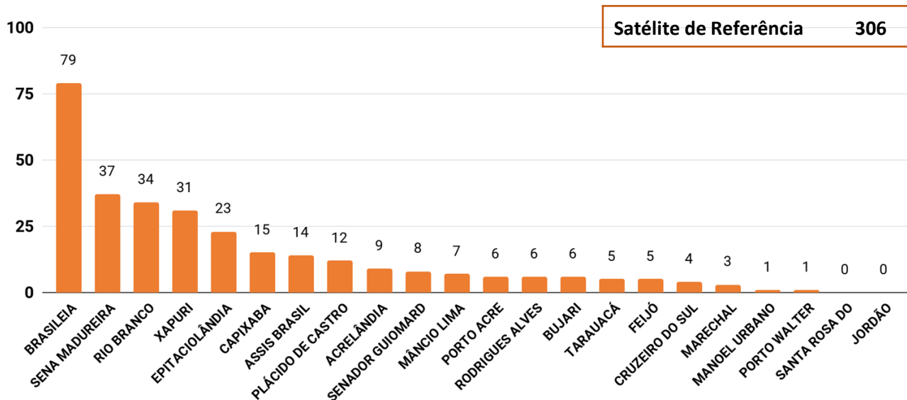
Figura 4 – Distribuição dos focos de queimadas acumulados no mês outubro de 01/10/2019 a 20/10/2019. (Satélite de referência AQUA TARDE)
