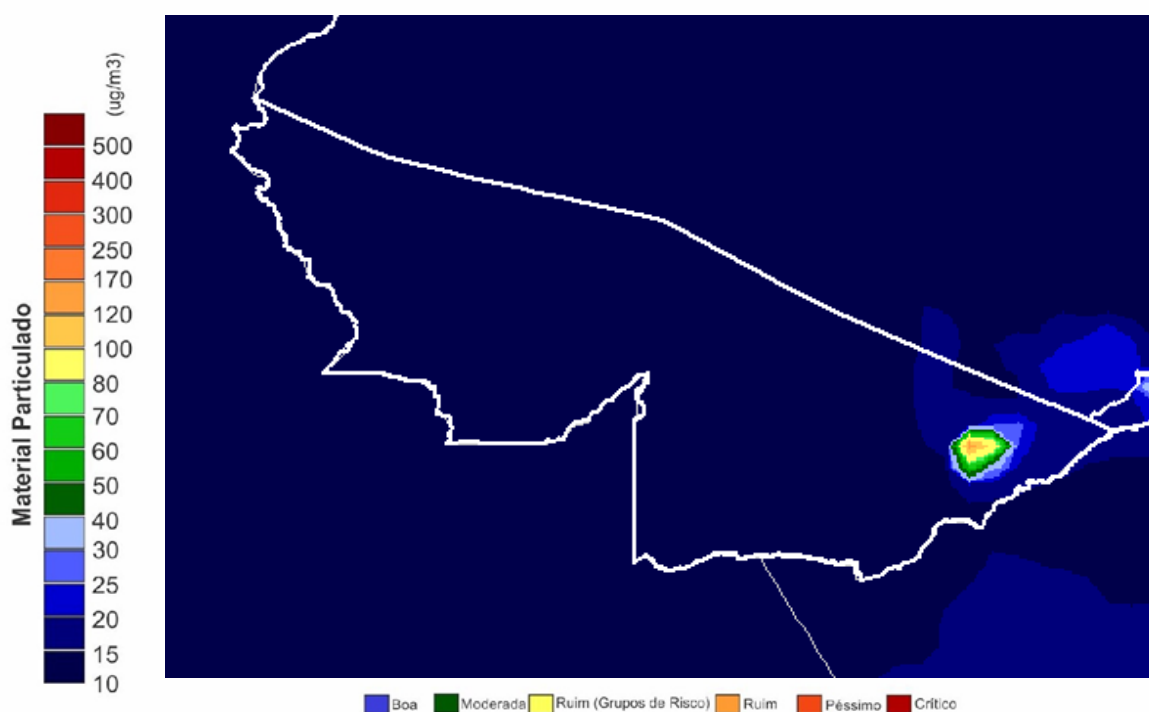
Figura 10 – Mapa de material Particulado CPTEC/INPE em 21/10/2019
