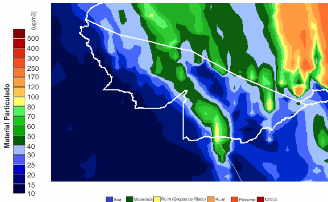
Figura 8 – Mapa de material Particulado CPTEC/INPE em 15/08/2019
