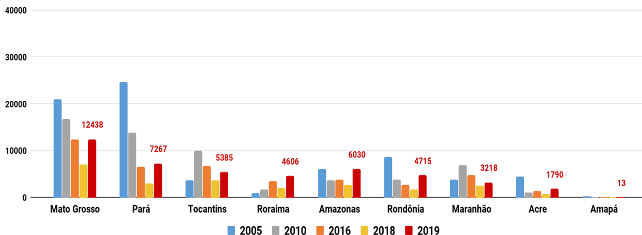
Figura 2 – Distribuição comparativa dos focos de queimadas acumulados de 01/08 a 14/08 na Amazônia legal, nos anos de 2005, 2010, 2016, 2018 e 2019 ( Satélite de Referência AQUA Tarde)
