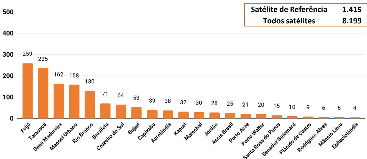
Figura 4 – Distribuição dos focos de queimadas acumulados no mês Agosto de 01/08/2019 a 14/08/2019 . ( Satélite de referência AQUA_M-T)
