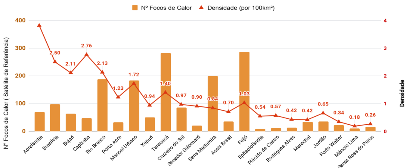
Figura 6 – Ocorrência de focos de queimadas e densidade por km 2 , por município em 01/01/2019 a 14/08/2019 ( Satélite de referência AQUA_M-T)
