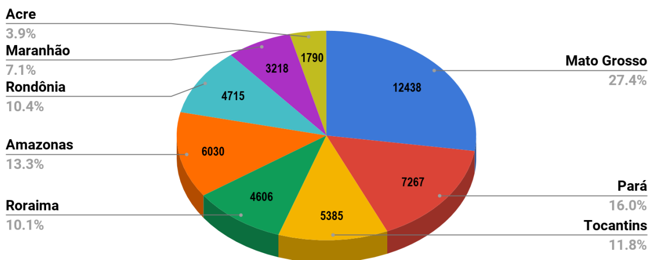
Figura 1 – Distribuição percentual dos focos de queimadas acumulados em 01/01/2019 a 14/08/2019 na Amazônia legal ( Satélite de Referência AQUA Tarde)
