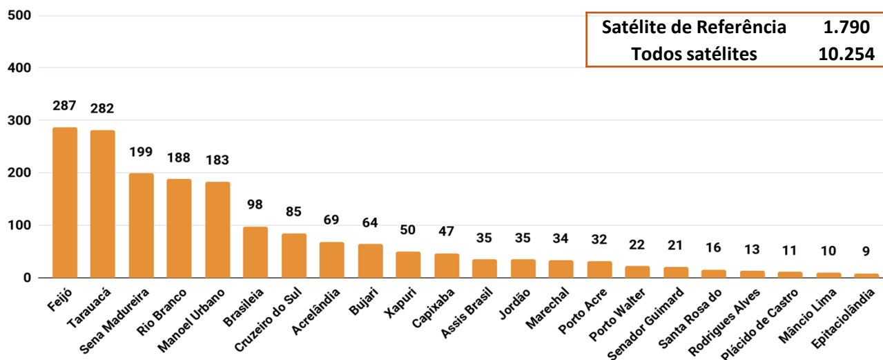
Figura 3 – Distribuição dos focos de queimadas acumulados de 01/01/2019 a 14/08/2019 , no Estado do Acre. ( Satélite de referência AQUA_M-T)
