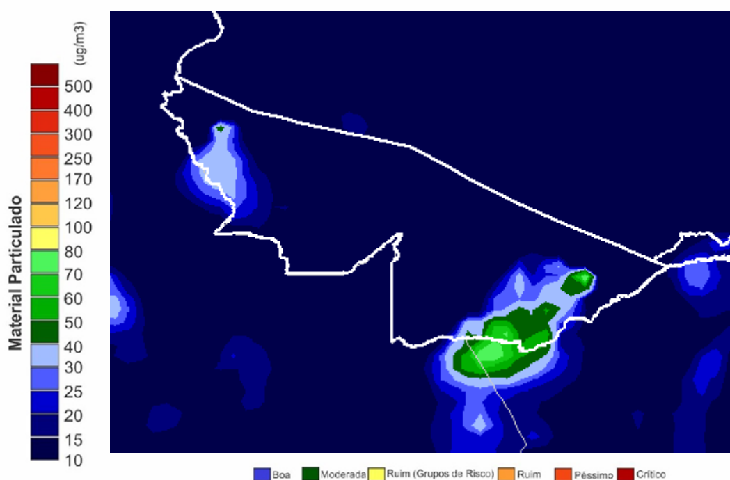
Figura 13 – Mapa de material Particulado CPTEC/INPE em 04.10.2018
