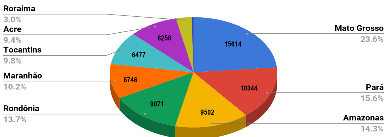
Figura 4 – Distribuição percentual dos focos de calor acumulados em 01/01/2018 a 03/10/2017 na Amazônia legal ( Satélite de Referência AQUA Tarde)
