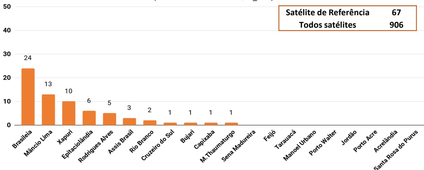
Figura 7 – Distribuição dos focos de calor acumulados no mês de 01/09/2018 a 03/10/2018 ( Satélite de referência AQUA_M-T)
