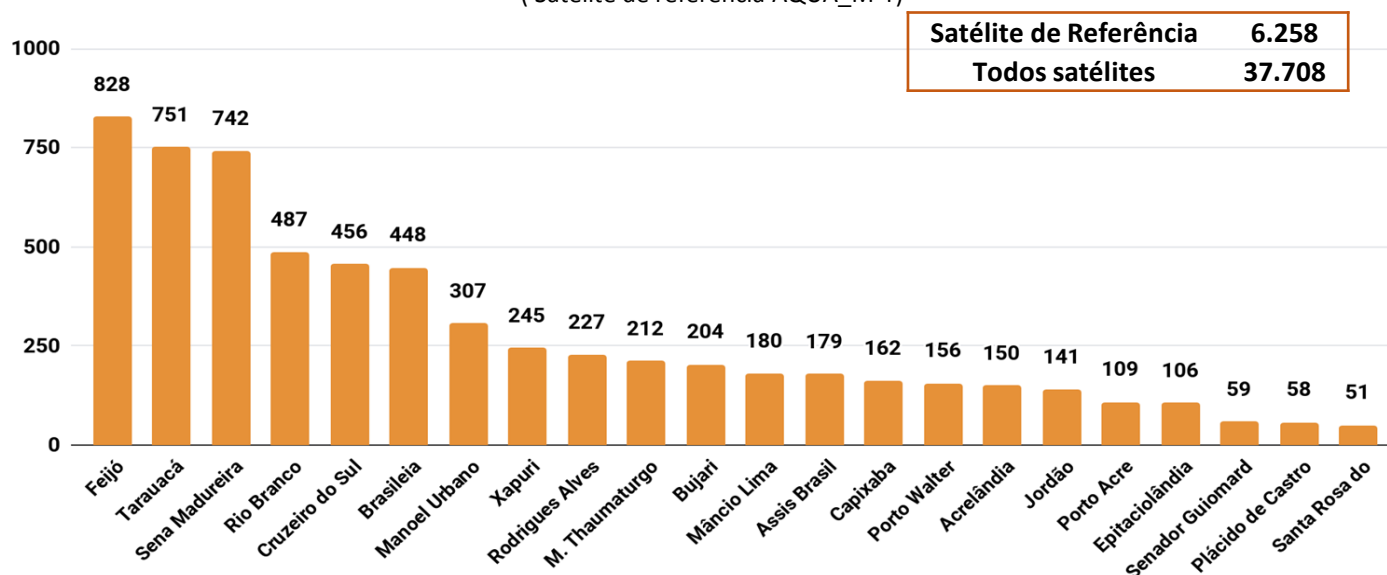
Figura 6 – Distribuição dos focos de calor acumulados de 01/01/2018 a 03/10/2018 , no Estado do Acre, segundo ( Satélite de referência AQUA_M-T)
