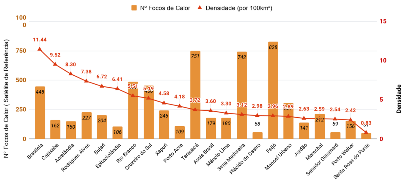
Figura 9 – Ocorrência de focos de calor e densidade por km 2 , por município em 01/01/2018 a 03/10/2018 ( Satélite de referência AQUA_M-T)
