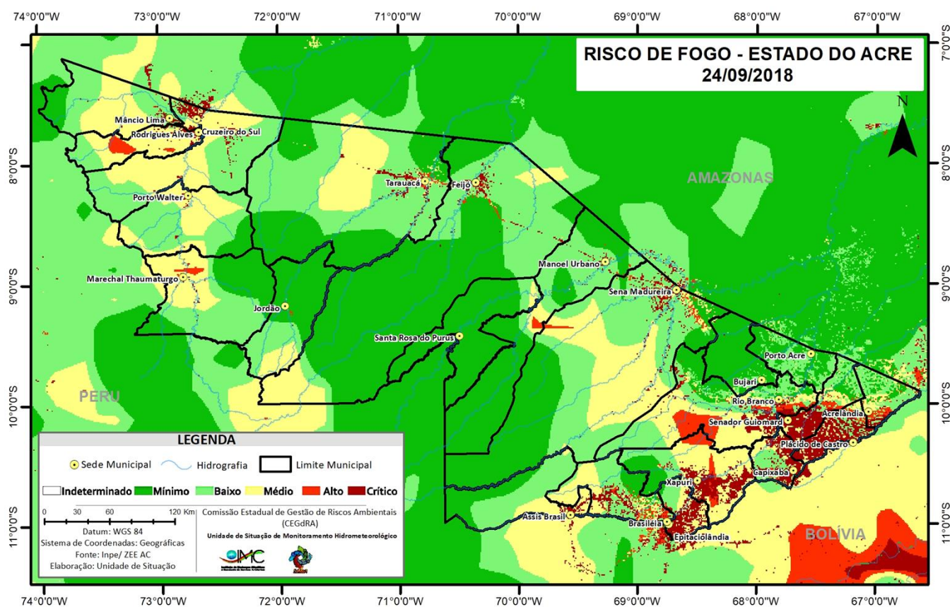
Figura 11 – Risco de Fogo para o estado do Acre em 24/09/2018
