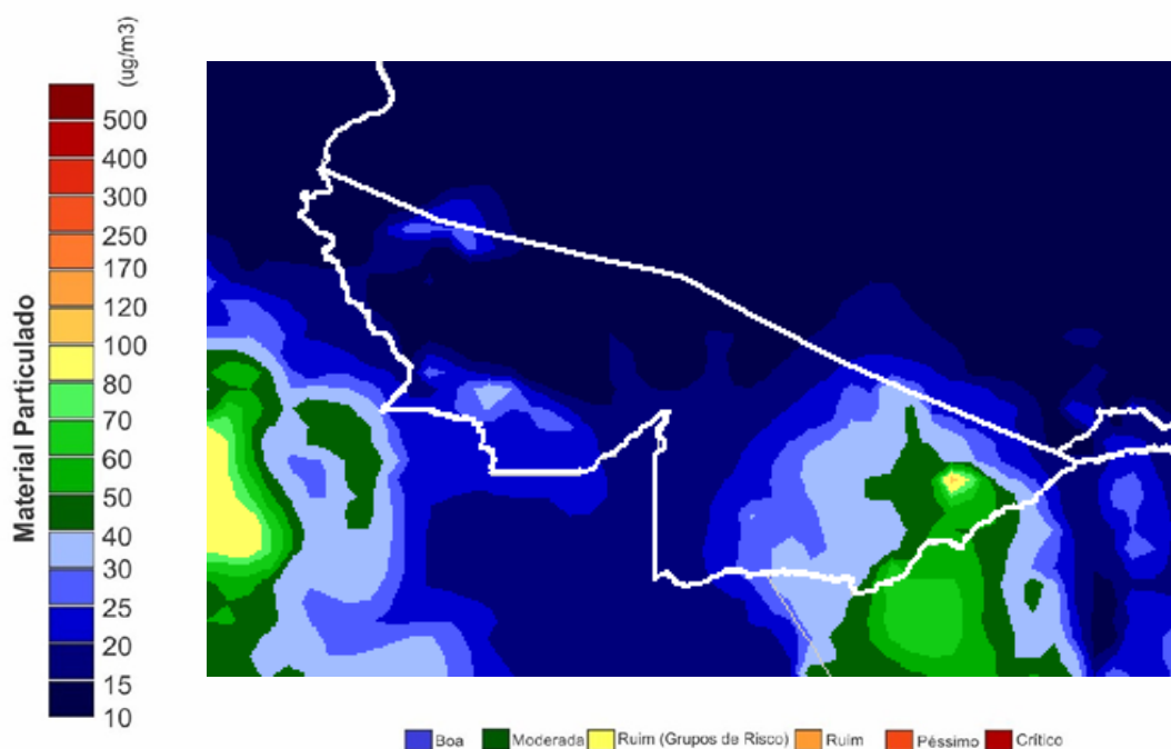
Figura 14 – Mapa de material Particulado CPTEC/INPE em 24.09.2018
