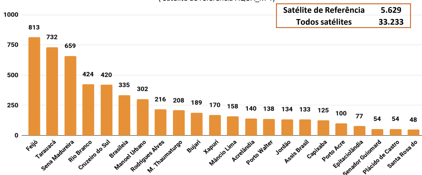
Figura 6 – Distribuição dos focos de calor acumulados de 01/01/2018 a 23/09/2018 , no Estado do Acre, segundo (Satélite de referência AQUA_M-T)
