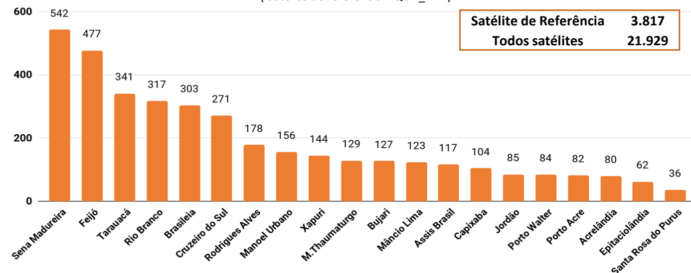
Figura 7 – Distribuição dos focos de calor acumulados no mês de 01/09/2018 a 23/09/2018 (Satélite de referência AQUA_M-T)
