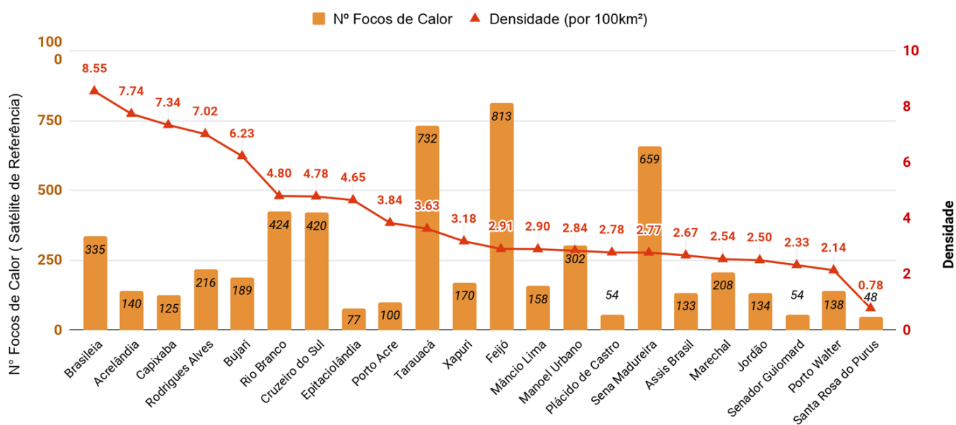
Figura 9 – Ocorrência de focos de calor e densidade por km 2 , por município em 01/01/2018 a 23/09/2018 ( Satélite de referência AQUA_M-T)
