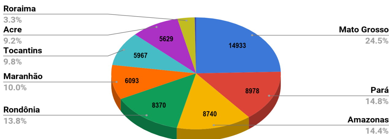
Figura 4 – Distribuição percentual dos focos de calor acumulados em 01/01/2018 a 23/09/2017 na Amazônia legal ( Satélite de Referência AQUA Tarde)
