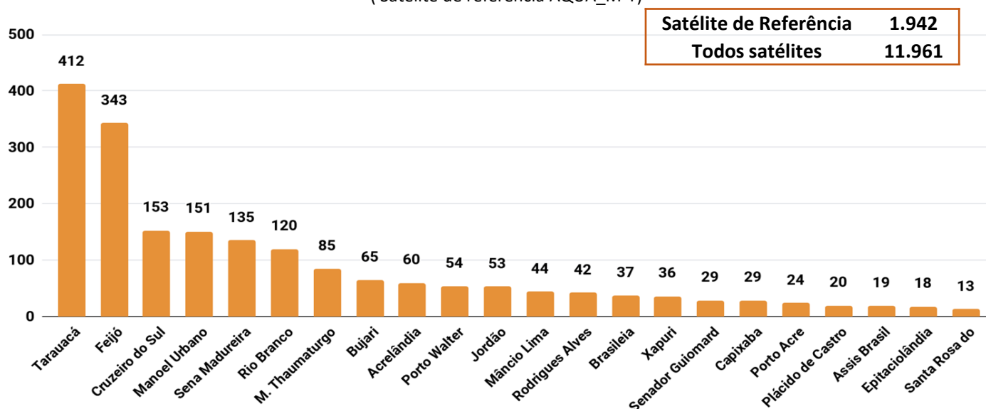
Figura 6 – Distribuição dos focos de calor acumulados de 01/01/2018 a 02/09/2018 , no Estado do Acre, segundo (Satélite de referência AQUA_M-T)
