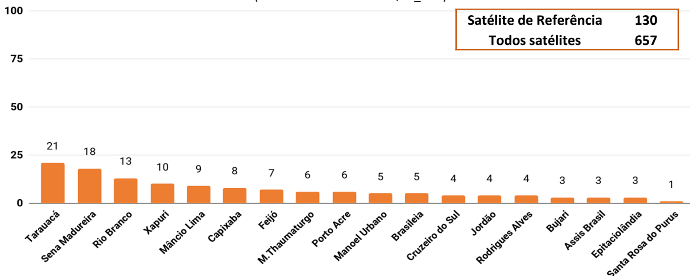
Figura 7 – Distribuição dos focos de calor acumulados no mês de 01/09/2018 a 02/09/2018 (Satélite de referência AQUA_M-T)
