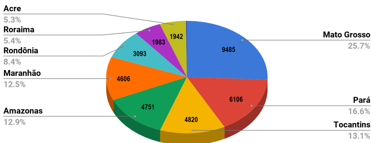
Figura 4 – Distribuição percentual dos focos de calor acumulados em 01/01/2018 a 02/09/2017 na Amazônia legal ( Satélite de Referência AQUA Tarde)
