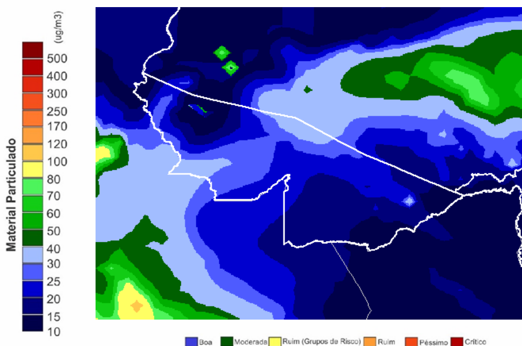
Figura 14 – Mapa de material Particulado CPTEC/INPE em 03.09.2018
