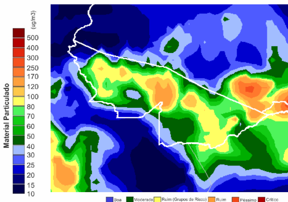
Figura 14 – Mapa de material Particulado CPTEC/INPE em 15.08.2018
