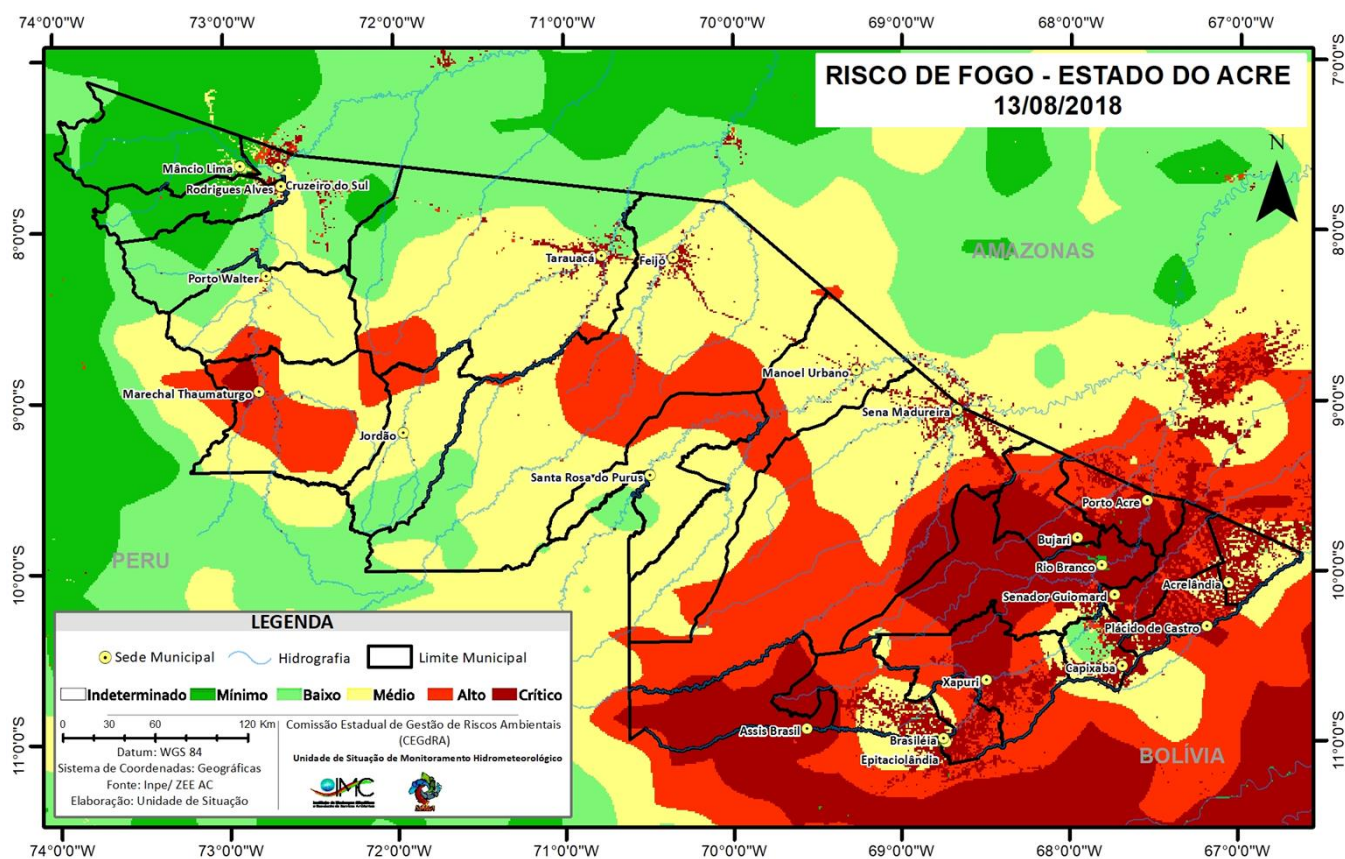
Figura 11 – Risco de Fogo para o estado do Acre em 13/08/2018
