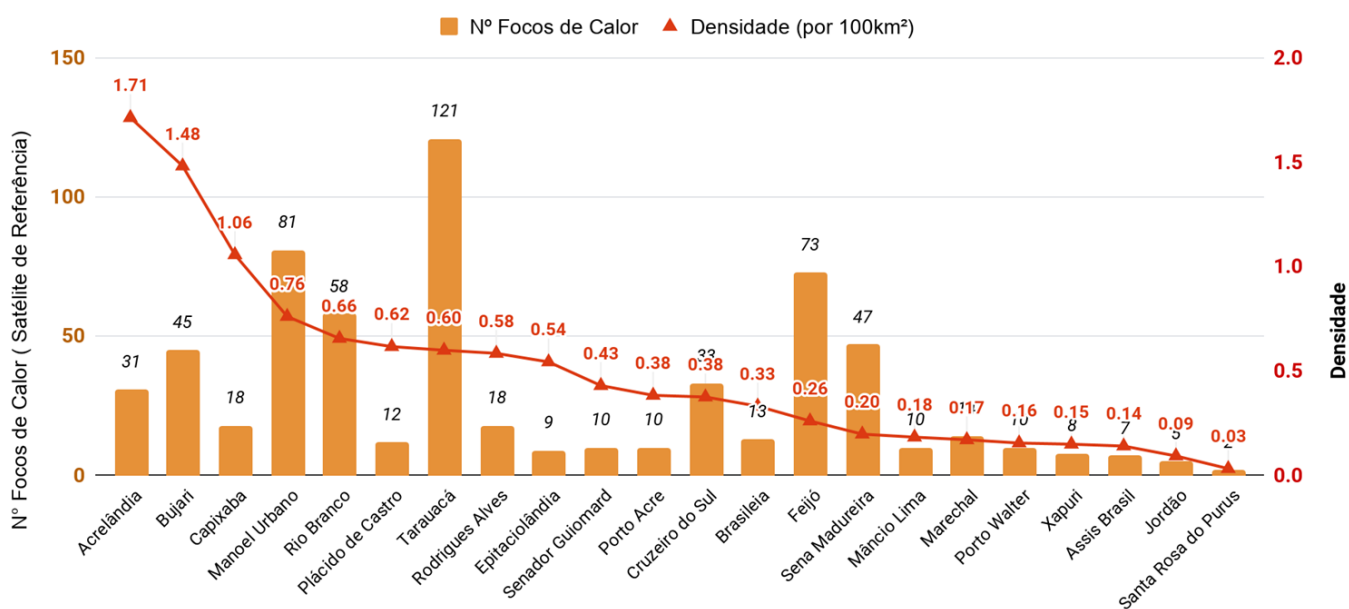
Figura 9 – Ocorrência de focos de calor e densidade por km 2 , por município em 01/01/2018 a 12/08/2018 ( Satélite de referência AQUA_M-T)
