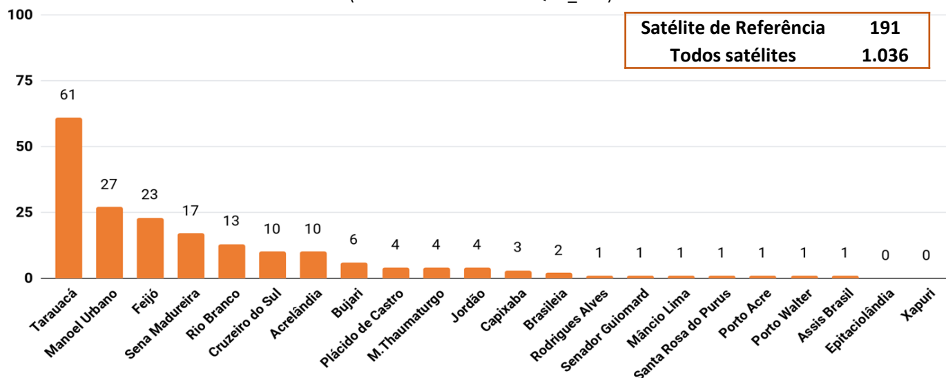
Figura 7 – Distribuição dos focos de calor acumulados no mês de 01.07.2018 a 12.08.2018 (Satélite de referência AQUA_M-T)
