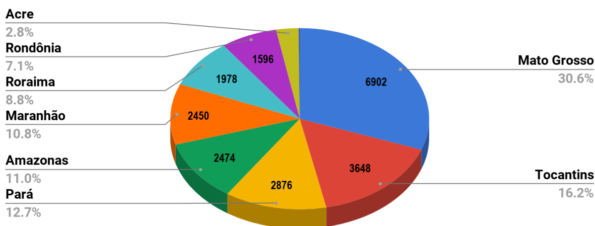
Figura 4 – Distribuição percentual dos focos de calor acumulados em 01.01.2018 a 12.08.2017 na Amazônia legal ( Satélite de Referência AQUA Tarde)
