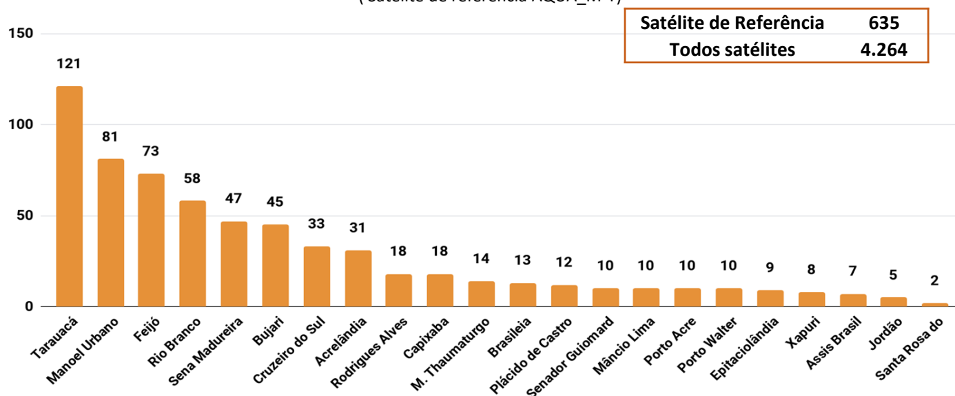
Figura 6 – Distribuição dos focos de calor acumulados de 01/01/2018 a 12/08/2018 , no Estado do Acre, segundo (Satélite de referência AQUA_M-T)
