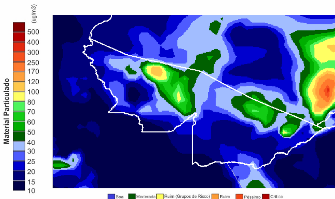
Figura 14 – Mapa de material Particulado CPTEC/INPE em 13.08.2018
