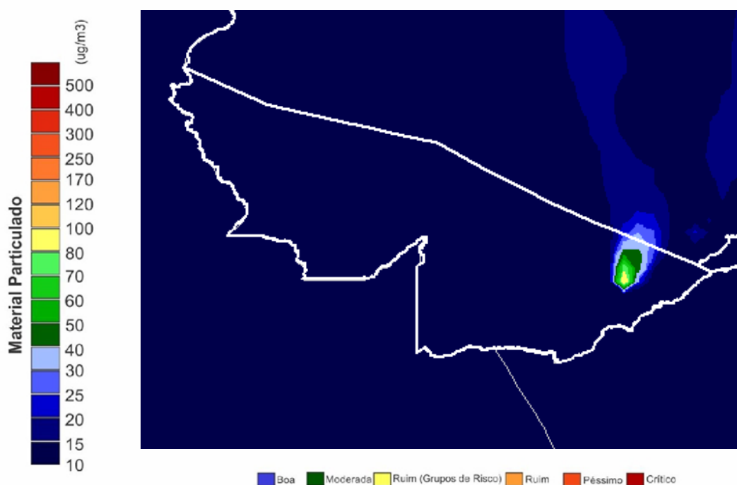
Figura 13 – Mapa de material Particulado CPTEC/INPE em 07.08.2018
