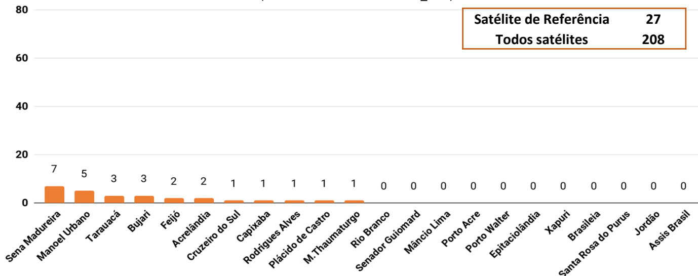
Figura 7 – Distribuição dos focos de calor acumulados no mês de 01.07.2018 a 06.08.2018 (Satélite de referência AQUA_M-T)
