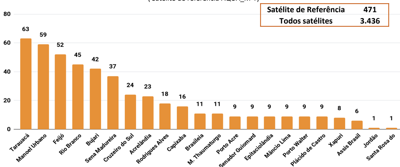
Figura 6 – Distribuição dos focos de calor acumulados de 01/01/2018 a 06/08/2018 , no Estado do Acre, segundo (Satélite de referência AQUA_M-T)
