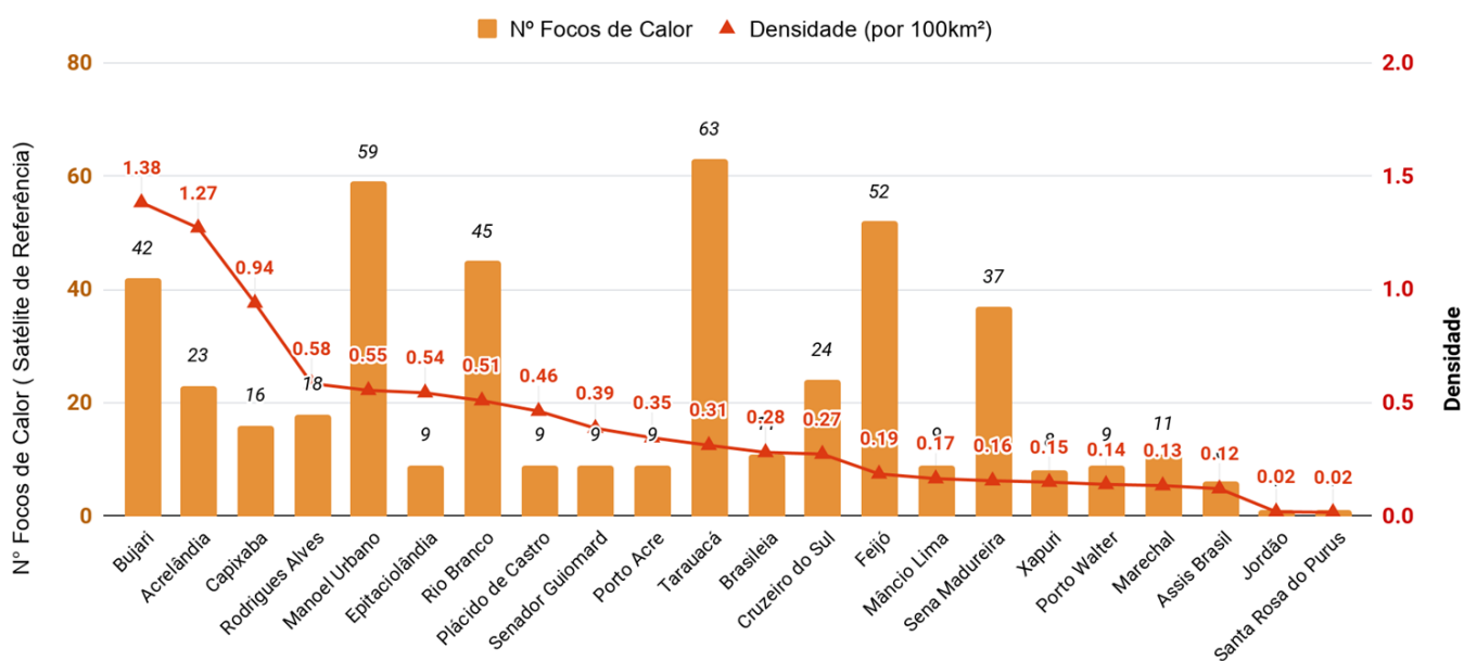
Figura 9 – Ocorrência de focos de calor e densidade por km 2 , por município em 01/01/2018 a 06/08/2018 ( Satélite de referência AQUA_M-T)
