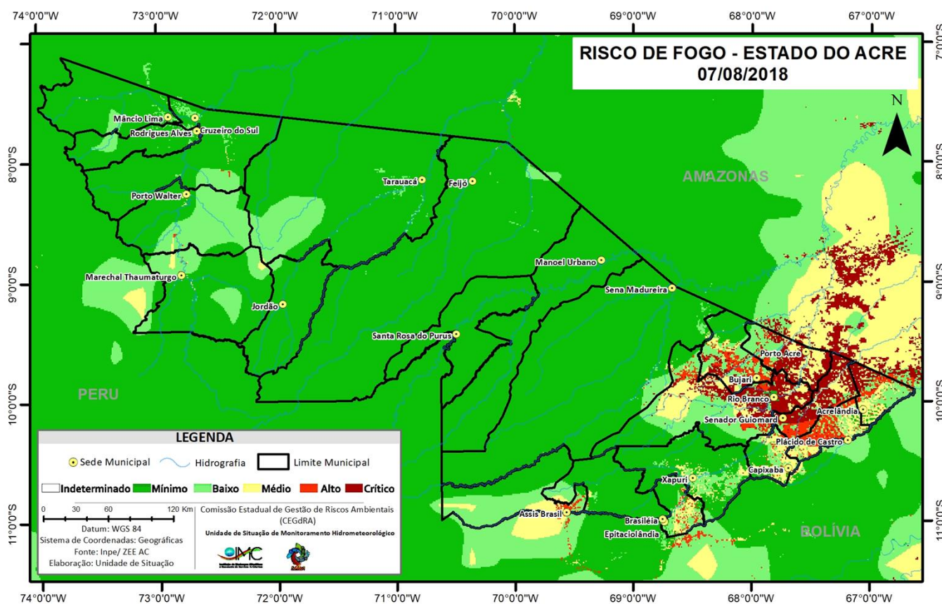
Figura 11 – Risco de Fogo para o estado do Acre em 07/08/2018
