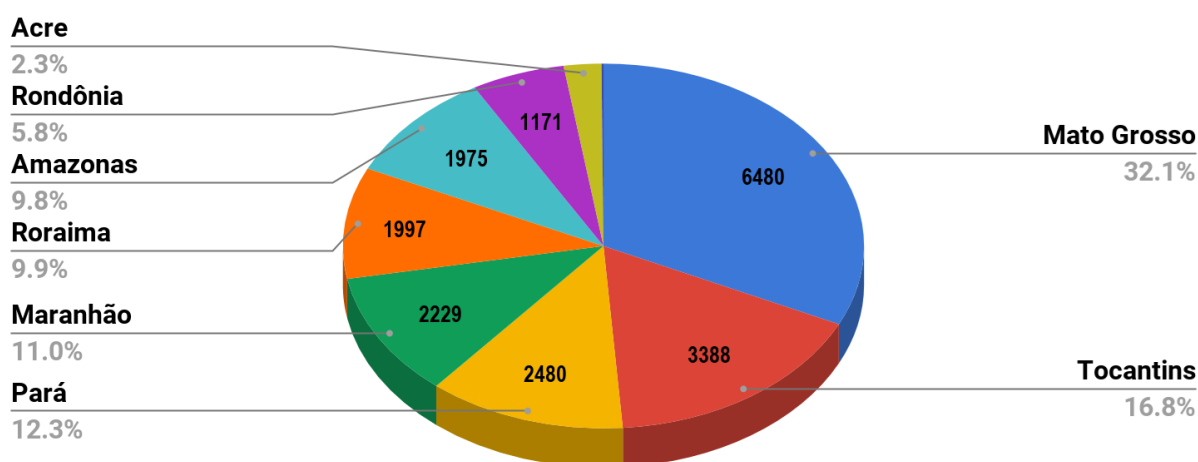
Figura 4 – Distribuição percentual dos focos de calor acumulados em 01.01.2018 a 06.08.2017 na Amazônia legal ( Satélite de Referência AQUA Tarde)
