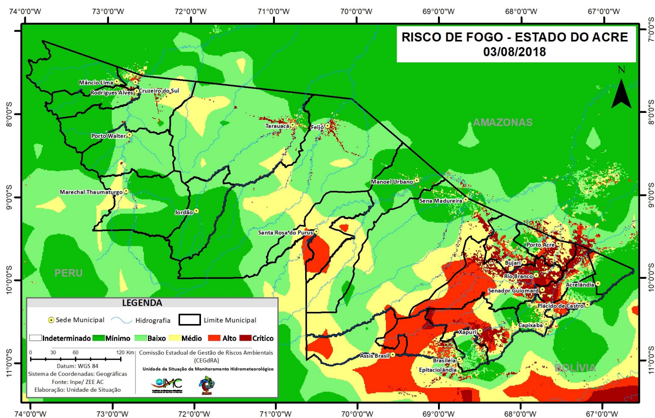
Figura 12 – Risco de Fogo para o estado do Acre em 03/08/2018
