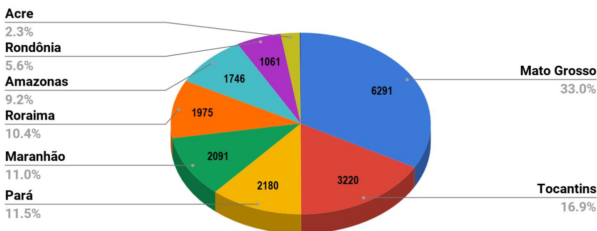
Figura 4 – Distribuição percentual dos focos de calor acumulados em 01.01.2018 a 02.08.2018 na Amazônia legal ( Satélite de Referência AQUA Tarde)
