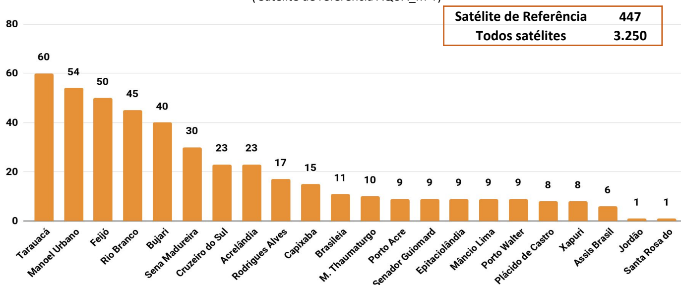
Figura 6 – Distribuição dos focos de calor acumulados de 01/01/2018 a 02/08/2018 , no Estado do Acre, segundo (Satélite de referência AQUA_M-T)
