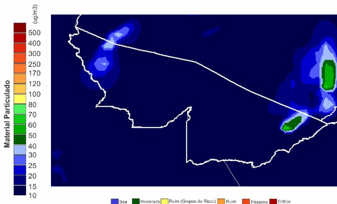
Figura 15 – Mapa de material Particulado CPTEC/INPE em 03.08.2018
