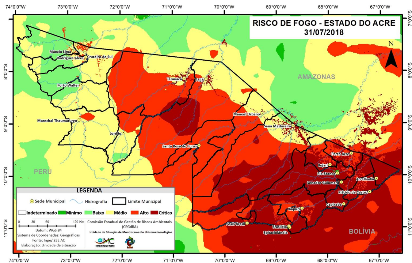
Figura 12 – Risco de Fogo para o estado do Acre em 31/07/2018
