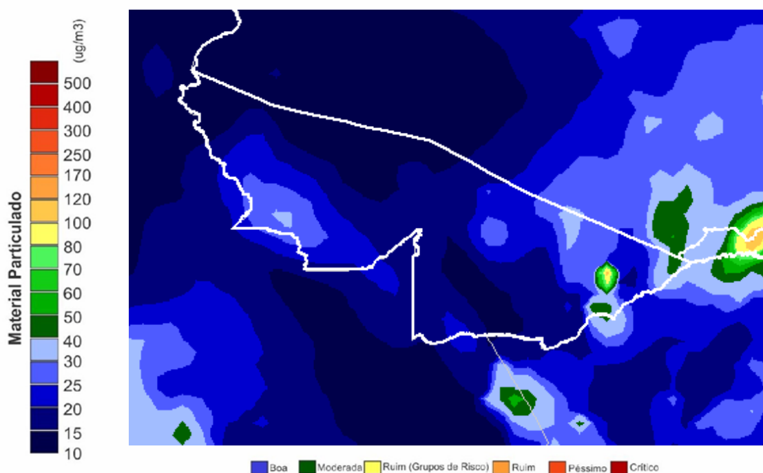
Figura 15 – Mapa de material Particulado CPTEC/INPE em 31.07.2018
