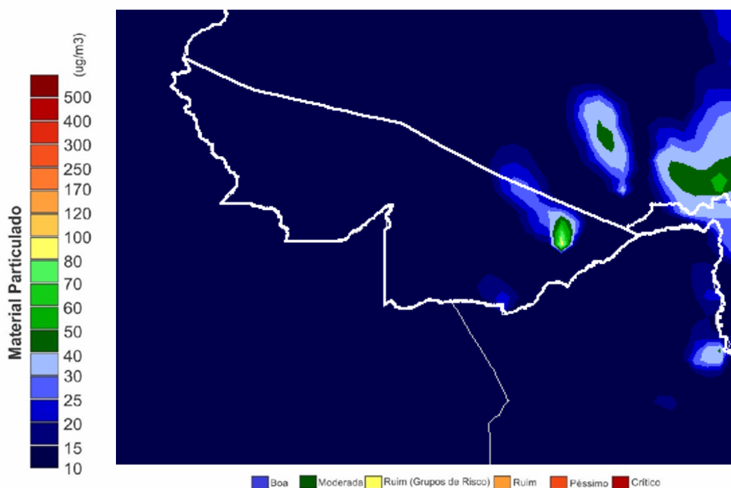
Figura 15 – Mapa de material Particulado CPTEC/INPE em 23.07.2018
