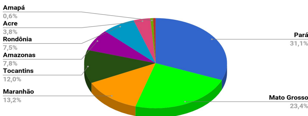
Figura 1 – Distribuição percentual dos focos de calor acumulados em 01.01.2017 a 22.11.2017 na Amazônia legal ( Satélite de Referência)
