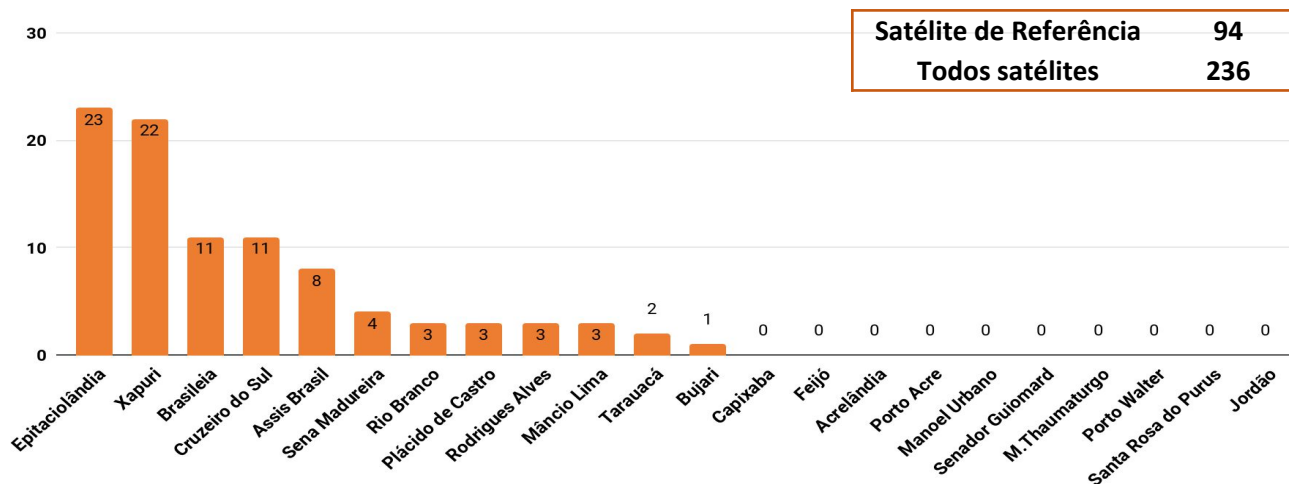
Figura 4 – Distribuição dos focos de calor acumulados no mês de 01.11.2017 a 22.11.2017 ( Satélite de Referência)
