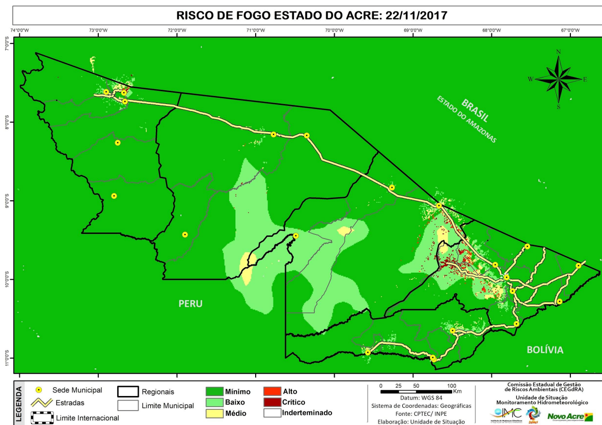
Figura 9 – Risco de Fogo para o estado do Acre em 22.11.2017/INPE-Proarco
