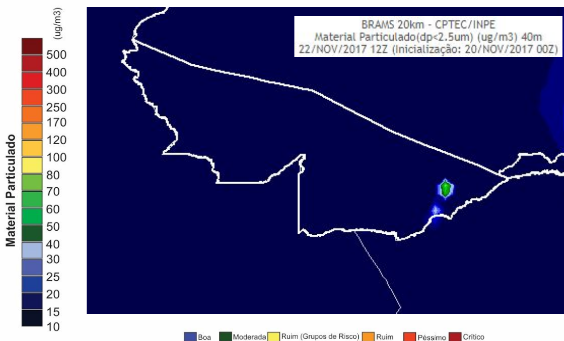
Figura 10– Mapa de material Particulado CPTEC/INPE em 22.11.2017.
