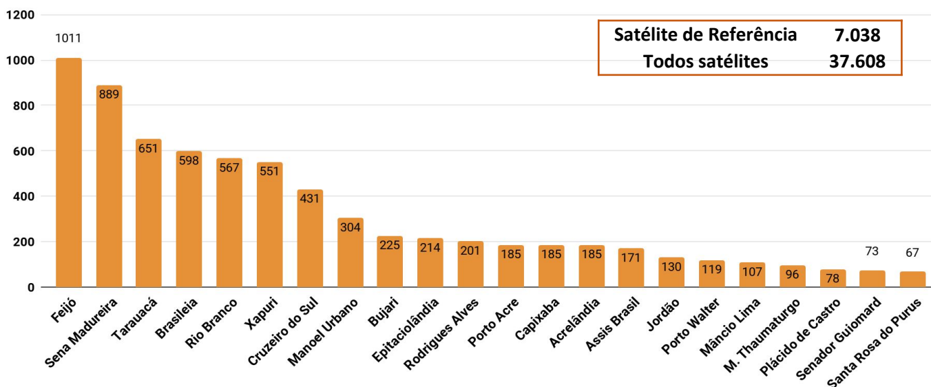
Figura 3 – Distribuição dos focos de calor acumulados em 01.01.2017 a 22.11.2017 no Estado ( Satélite de Referência)
