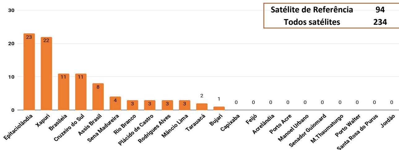
Figura 4 – Distribuição dos focos de calor acumulados no mês de 01.11.2017 a 21.11.2017 ( Satélite de Referência)
