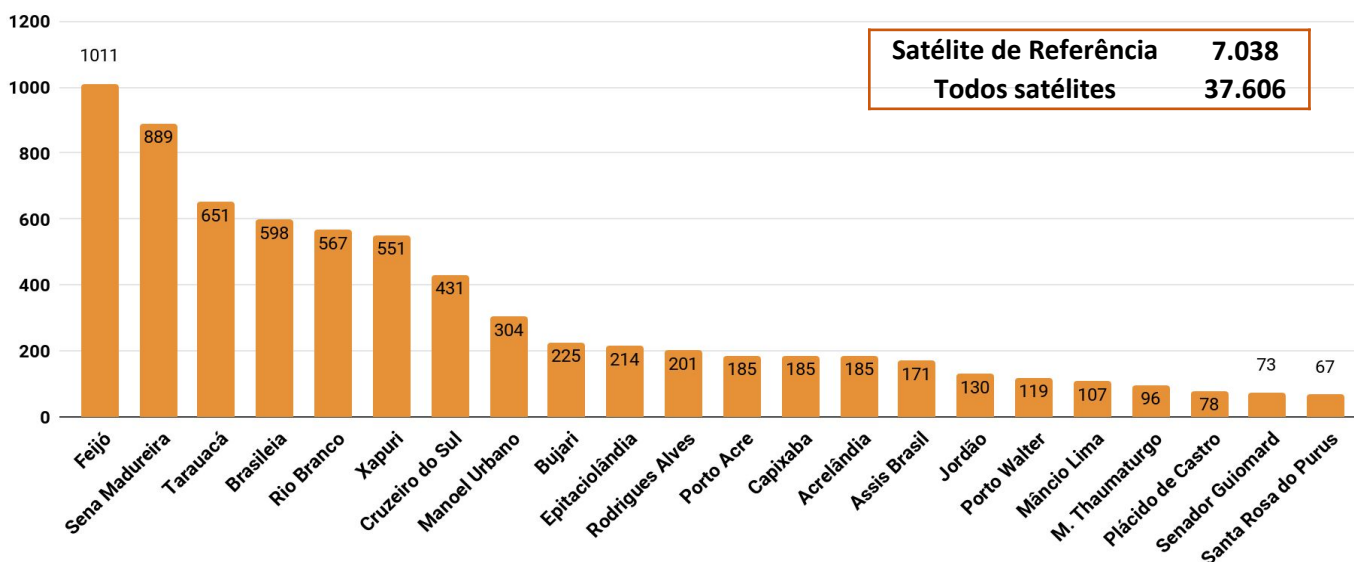
Figura 3 – Distribuição dos focos de calor acumulados em 01.01.2017 a 21.11.2017 no Estado ( Satélite de Referência)
