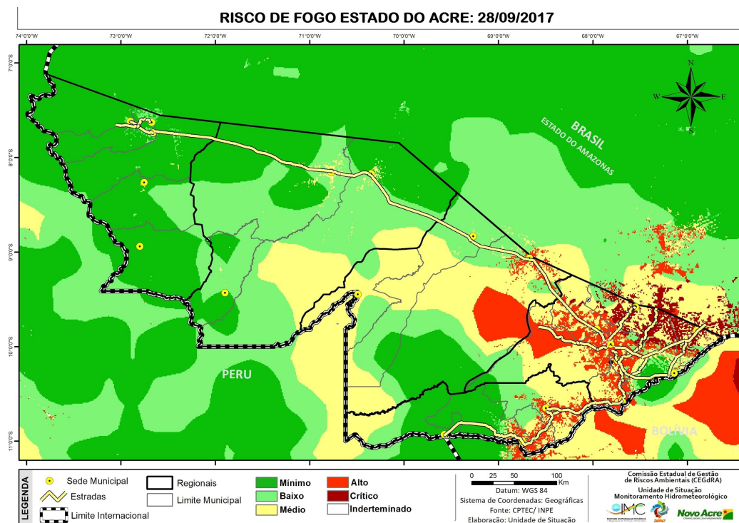
Figura 7 – Risco de Fogo para o estado do Acre em 28.09.2017/INPE-Proarco
