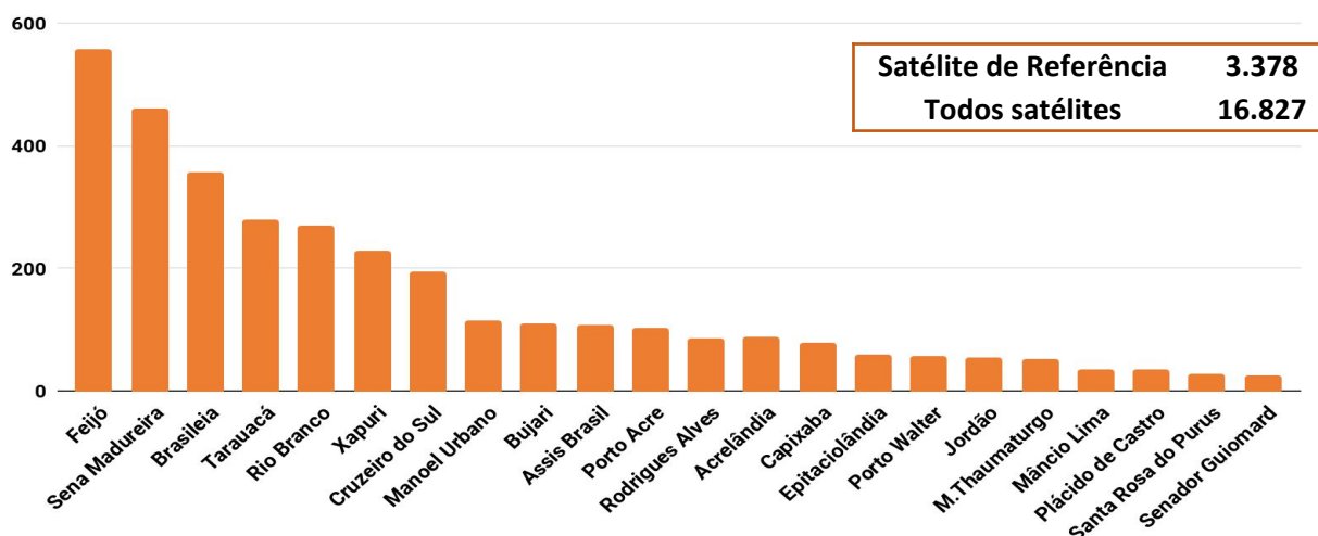
Figura 4 – Distribuição dos focos de calor acumulados no mês de 01.09.2017 a 28.09.2017
