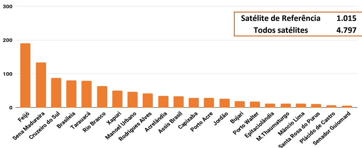
Figura 4 – Distribuição dos focos de calor acumulados no mês de 01.09.2017 a 11.09.2017
