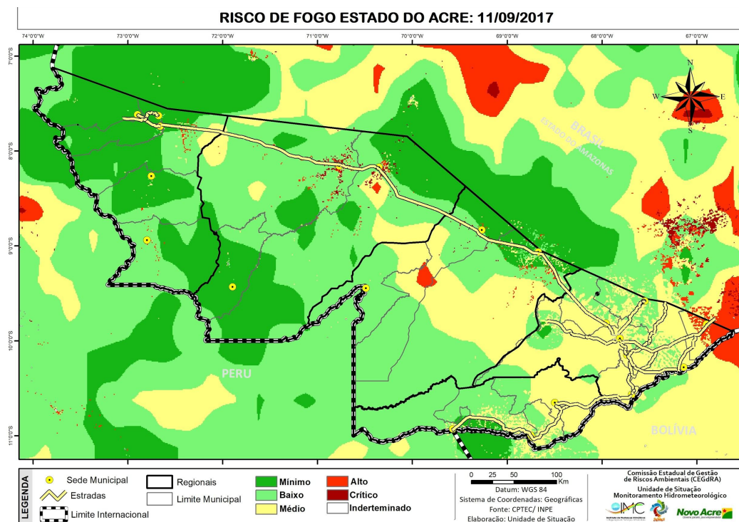
Figura 7 – Risco de Fogo para o estado do Acre em 11.09.2017/INPE-Proarco
