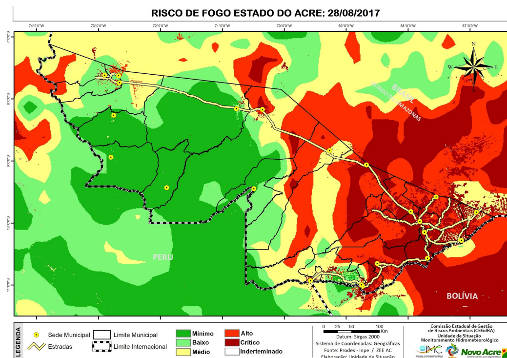
Figura 7 – Risco de Fogo para o estado do Acre em 28.08.2017/INPE-Proarco
