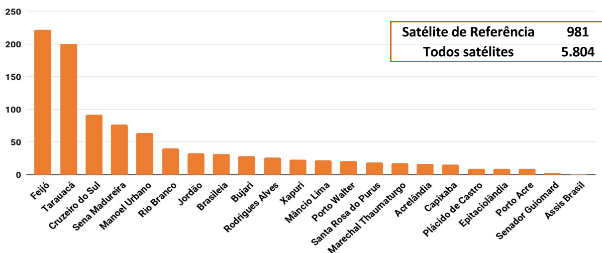
Figura 4 – Distribuição dos focos de calor acumulados no mês de 01.08.2017 a 28.08.2017
