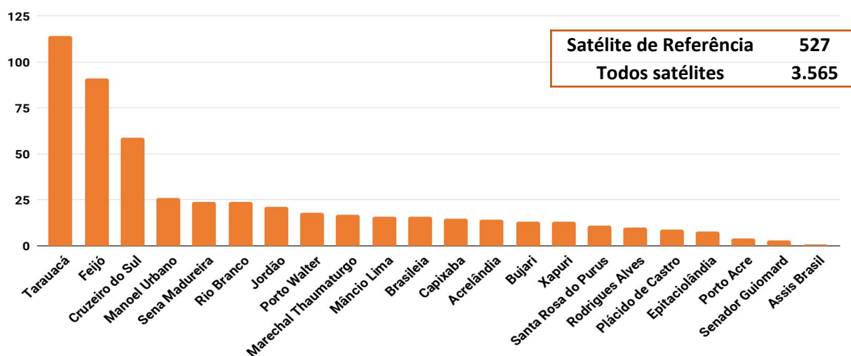
Figura 4 – Distribuição dos focos de calor acumulados no mês de 01.08.2017 a 23.08.2017
