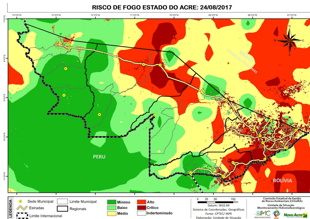
Figura 7 – Risco de Fogo para o estado do Acre em 24.08.2017/INPE-Proarco
