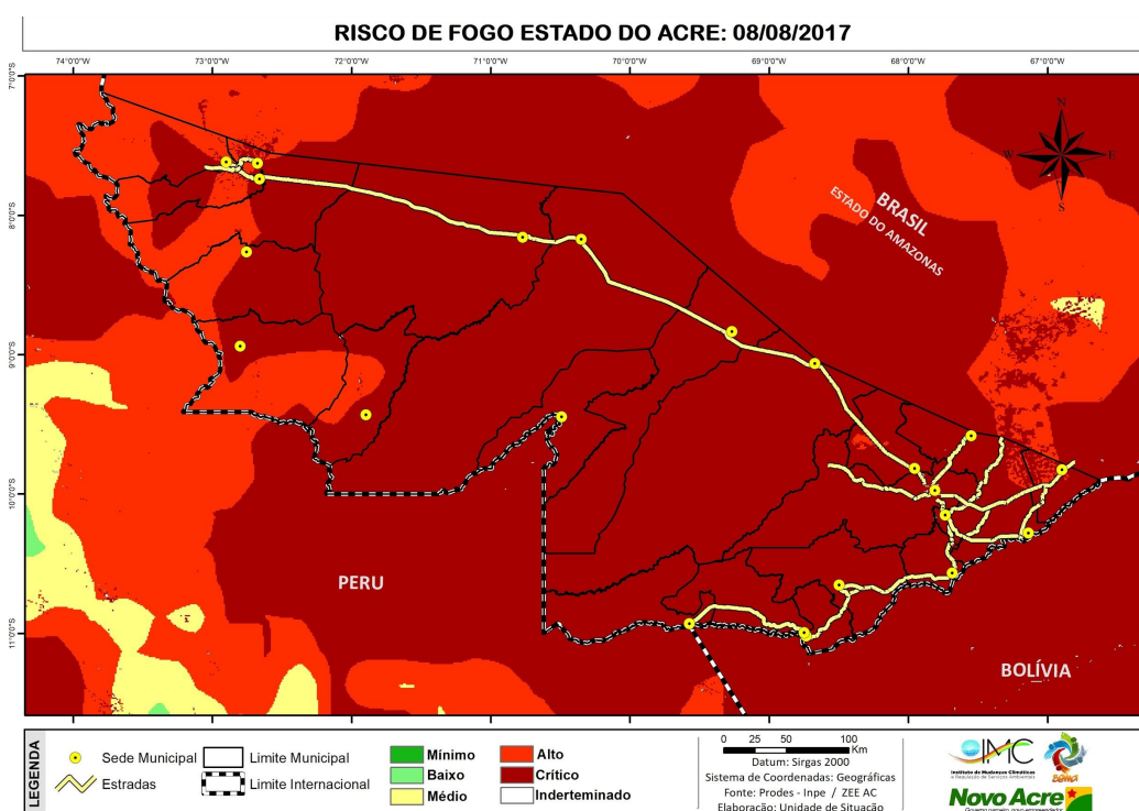
Figura 7 – Risco de Fogo para o estado do Acre em 08.08.2017/INPE-Proarco
