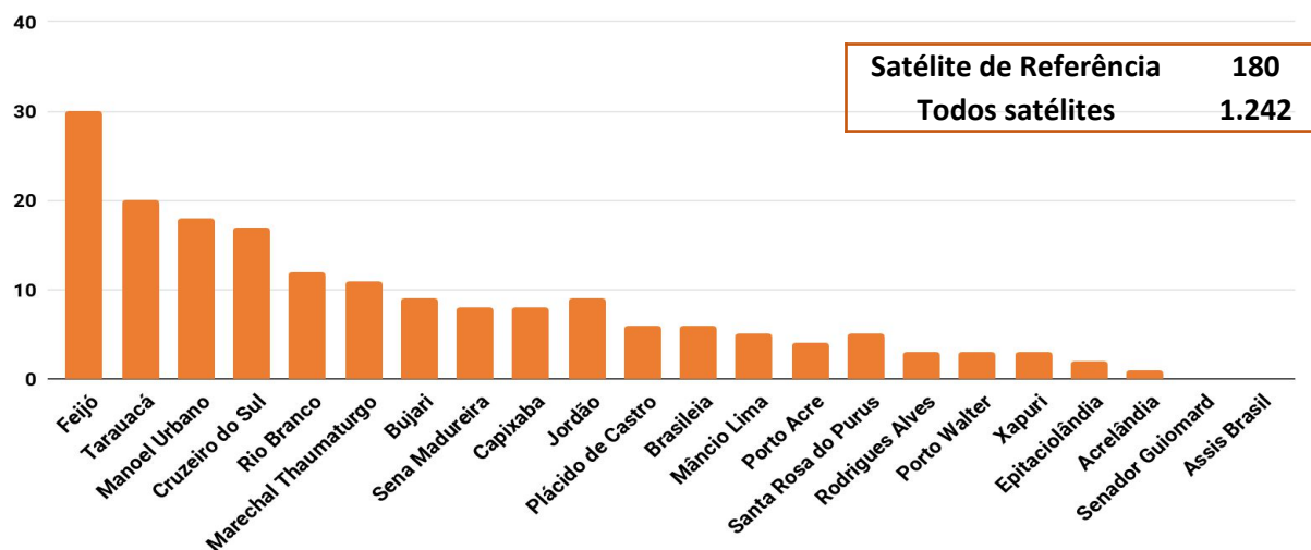
Figura 4 – Distribuição dos focos de calor acumulados no mês de 01.08.2017 a 08.08.2017
