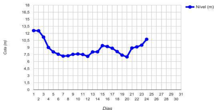
Cotograma Rio Envira (Feijó_Ponte) - Fevereiro/2017
