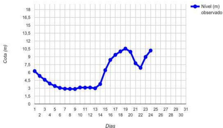
Cotograma Rio Acre (Capixaba) - Fevereiro/2017
