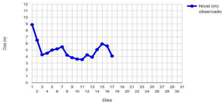
Cotograma Rio Liberdade (Cruzeiro do Sul_Ponte) - Fevereiro/2017
