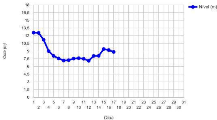
Cotograma Rio Envira (Feijó_Ponte) - Fevereiro/2017
