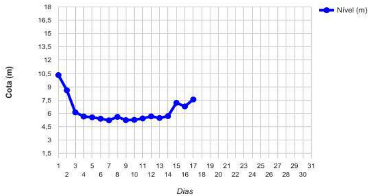
Cotograma Rio Purus (Manoel Urbano_Ponte) - Fevereiro/2017
