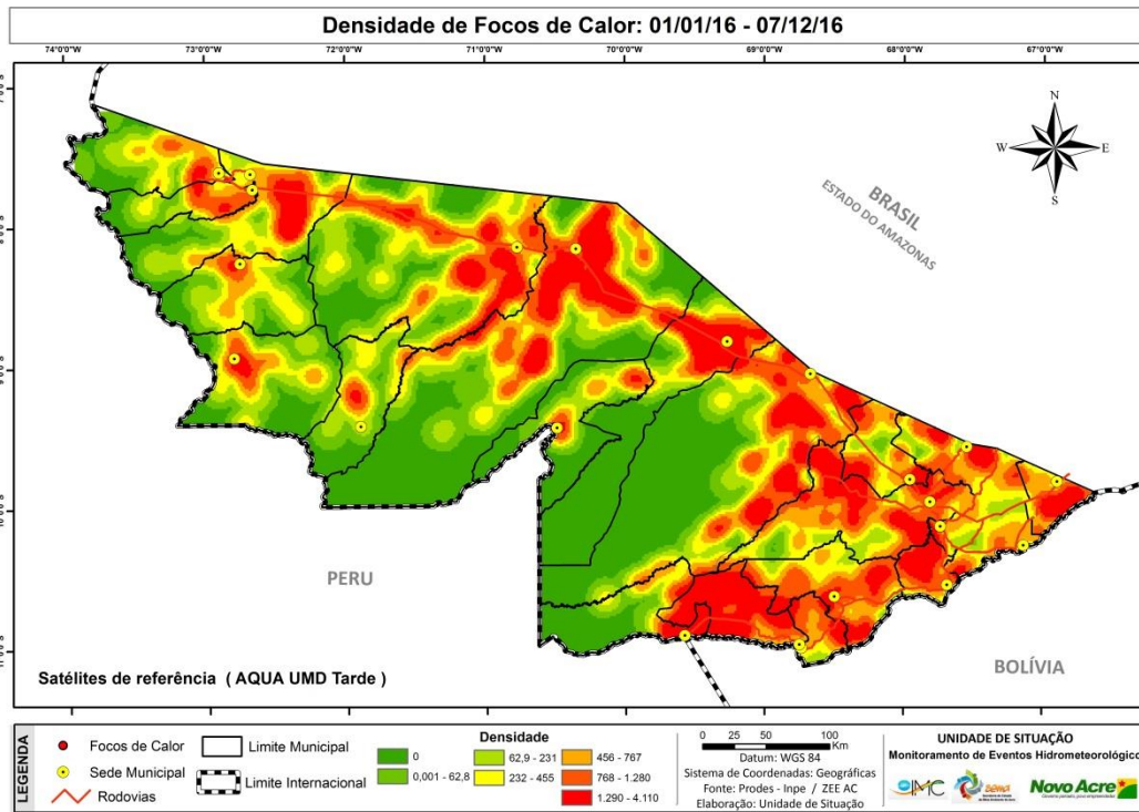
Figura 6 – Densidade dos focos de calor acumulados de 01.01.2016 a 07.12.2016
