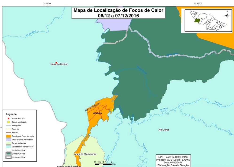
Figura 7 – Distribuição dos focos de calor no município de Marechal Thaumaturgo
