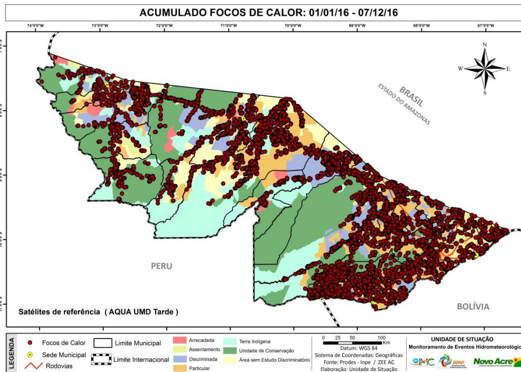
Figura 5 – Distribuição dos focos de calor acumulados de 01.01.2016 a 07.12.2016
