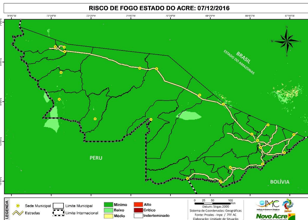
Figura 08 – Risco de Fogo para estado do Acre em 07.12.2016/INPE-Proarco
