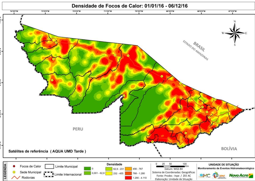
Figura 7 – Densidade dos focos de calor acumulados de 01.01.2016 a 06.12.2016
