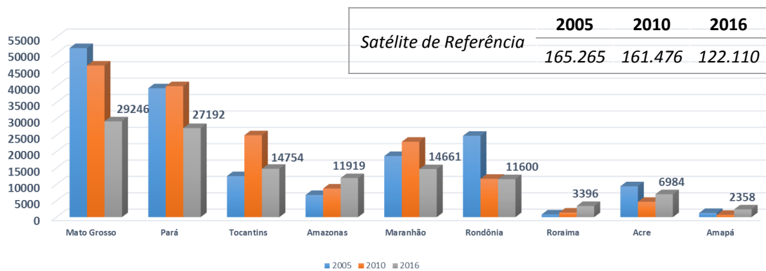
Figura 4 – Acumulado de focos de calor nos Estados da Amazônia Legal.
