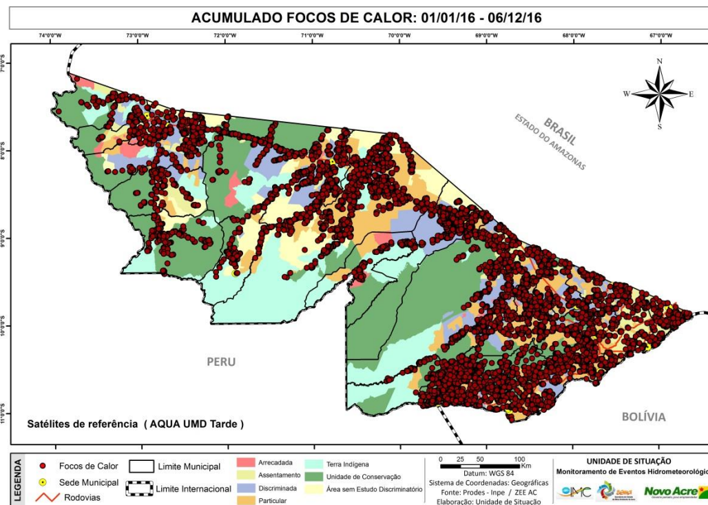
Figura 6 – Distribuição dos focos de calor acumulados de 01.01.2016 a 06.12.2016
