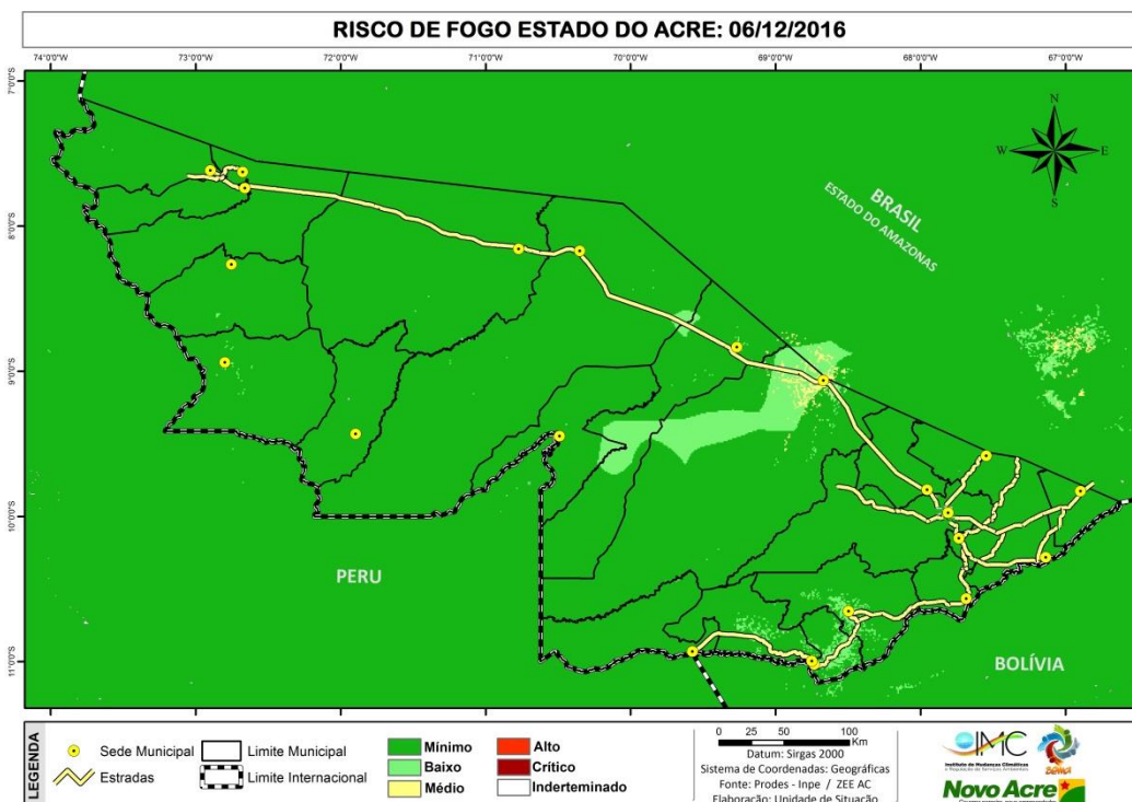
Figura 09 – Risco de Fogo para estado do Acre em 06.12.2016/INPE-Proarco
