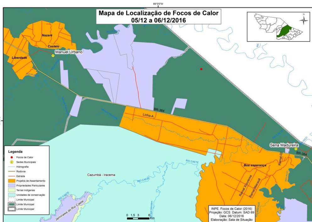
Figura 8 – Distribuição dos focos de calor no município de Sena Madureira
