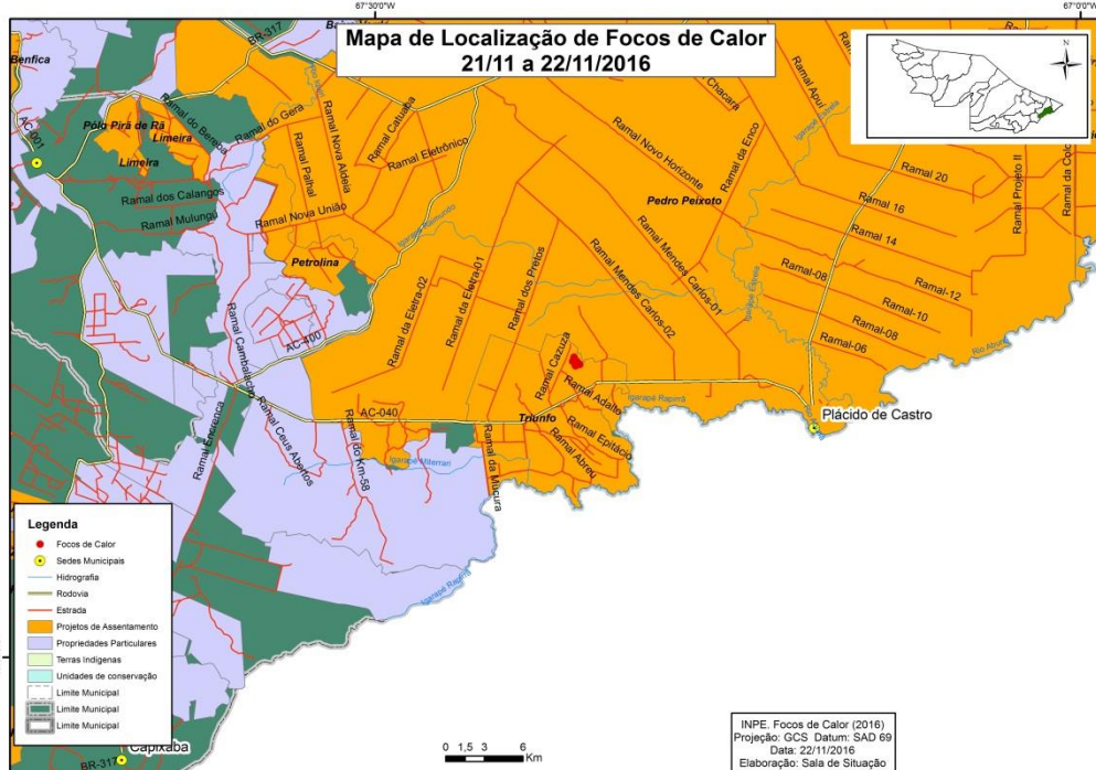
Figura 8 – Distribuição dos focos de calor no município de Plácido de Castro
