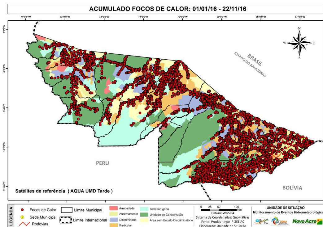
Figura 6 – Distribuição dos focos de calor acumulados de 01.01.2016 a 22.11.2016
