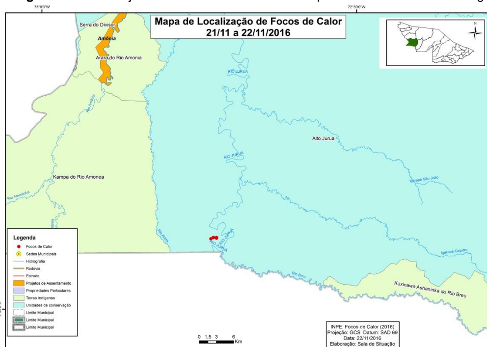
Figura 9 – Distribuição dos focos de calor no município de Marechal Thaumaturgo
