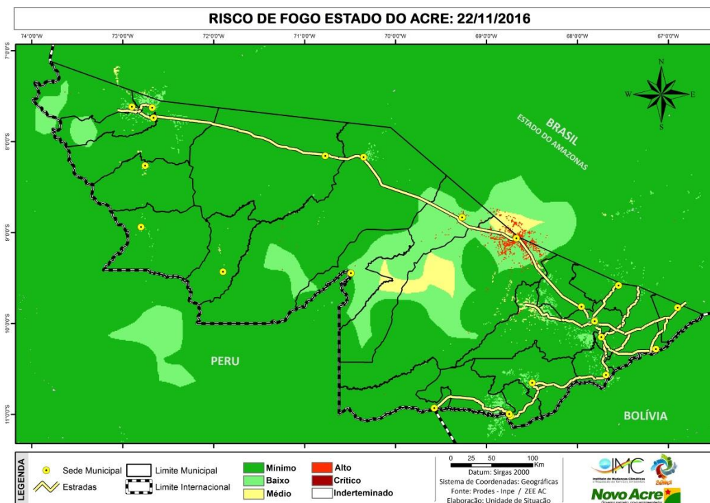
Figura 10 – Risco de Fogo para estado do Acre em 22.11.2016/INPE-Proarco
