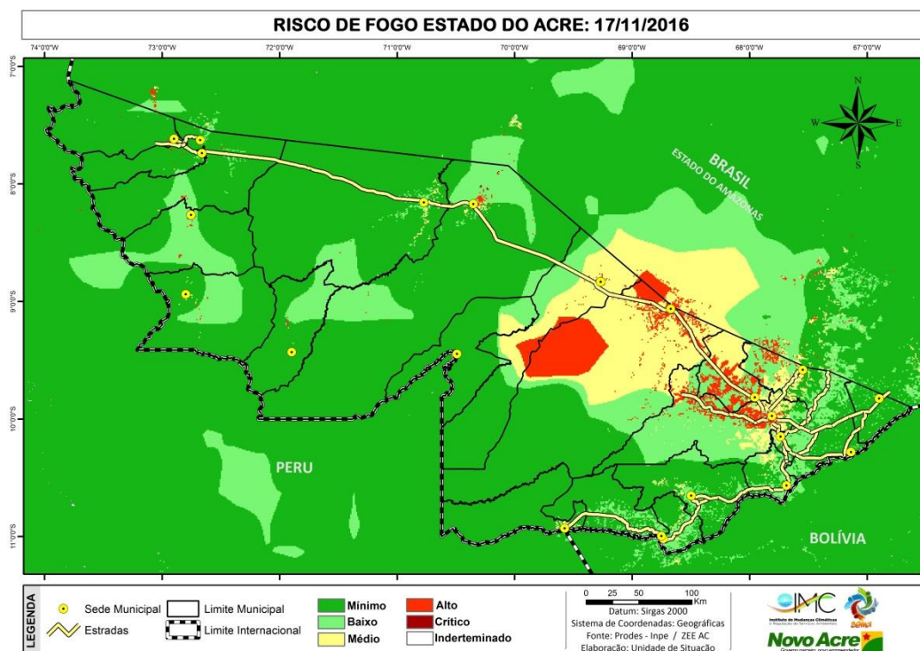
Figura 10 – Risco de Fogo para estado do Acre em 17.11.2016/INPE-Proarco
