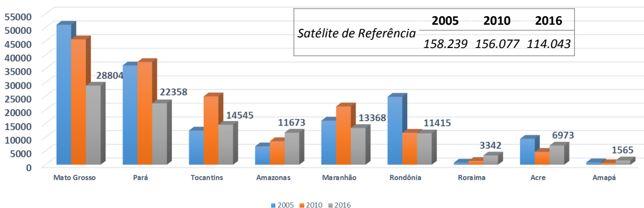
Figura 5 – Acumulado de focos de calor nos Estados da Amazônia Legal.
