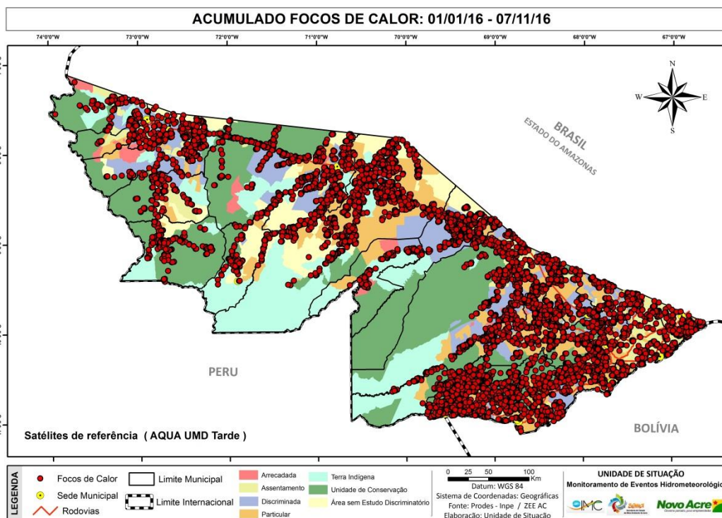
Figura 6 – Distribuição dos focos de calor acumulados de 01.01.2016 a 07.11.2016
