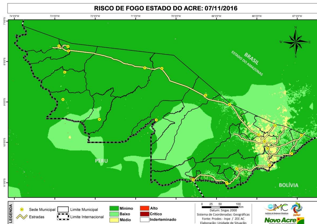
Figura 10 – Risco de Fogo para estado do Acre em 07.11.2016/INPE-Proarco
